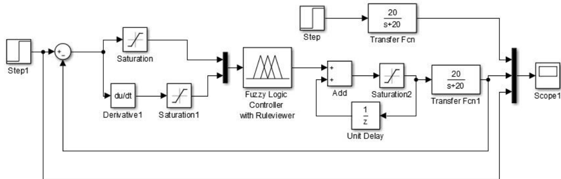
Figura 7 – Controlador Fuzzy incremental.
