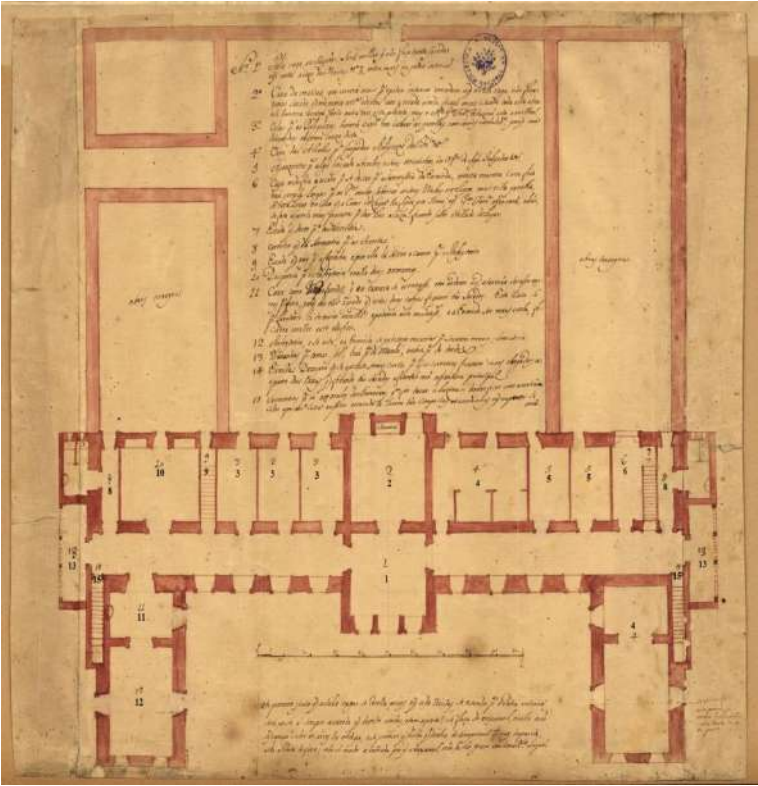
Fig. 1: Parte de planta do Convento Franciscano de Coimbra [ca 1755?]
